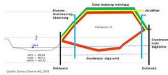
Schematische Darstellung, Sicherung der Altlast K20
